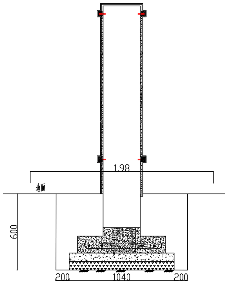
基础开挖断面图1
