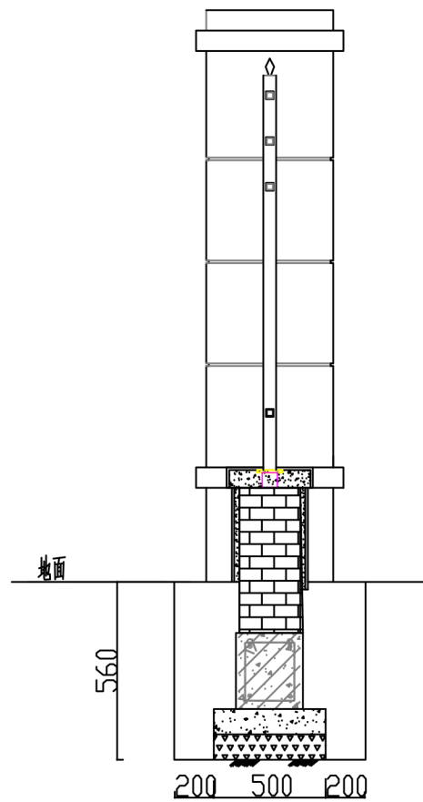
基础开挖断面图2
