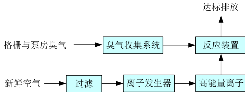
图 5.5-2 除臭工艺流程
