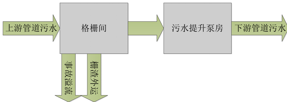
图 5.5-1 污水泵站工艺流程图
