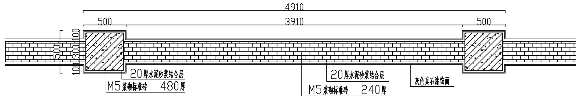
围墙标准横断面图
