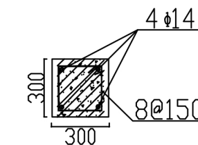
地梁基础图
