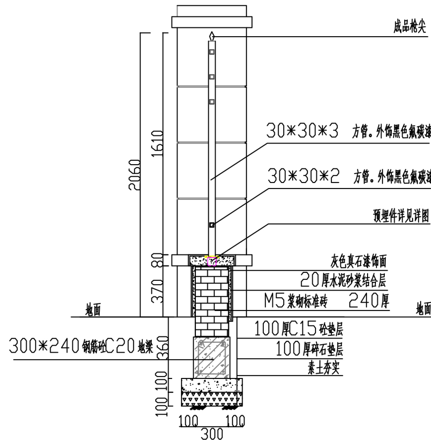
2-2 剖面图
