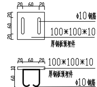
预埋件详图
